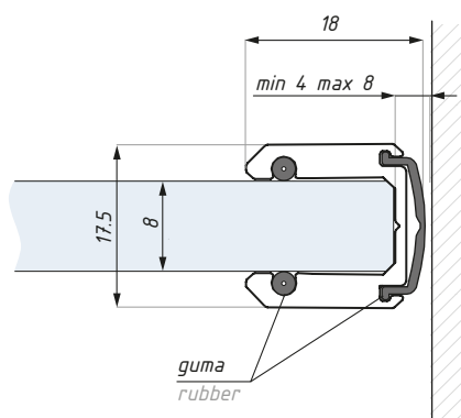
Mocowanie przy ścianie Wall montage
