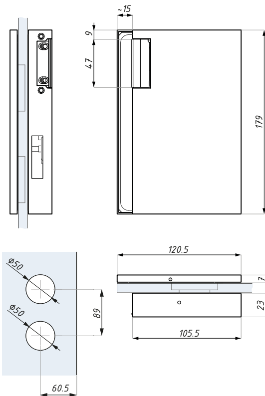
Przygotowanie szkła Glass preparation
