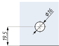
Wycięcie w szkłe dla szczeliny 5 mm Glass preparation: gap 5mm
