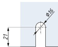
Wycięcie w szkłe dla szczeliny 0-5 mm Glass preparation: adjustments 0-5 mm
